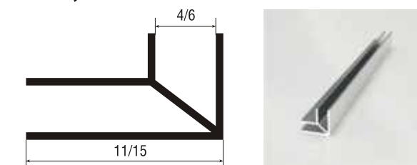
Планка угловая для щита (елочка)
