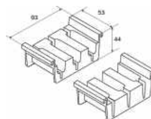
арт. 2056.51 Подставка для 3-х ножей для лотков Cuisio Aqua в ящик 400,500,800 мм
