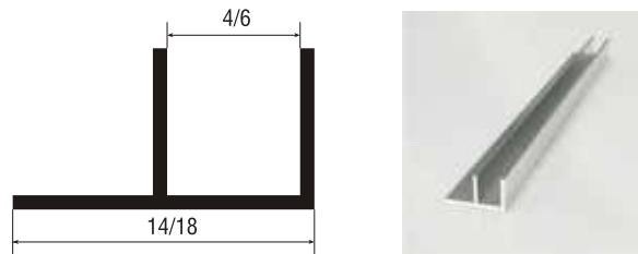
Планка угловая для щита
